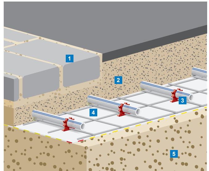
Beispielaufbau Uponor Meltaway Schnee- und Eisfreihaltung im Sandbett
