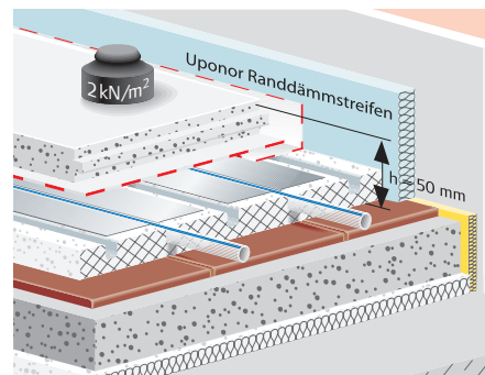
Uponor Siccus auf vorhandenem Altbelag.
