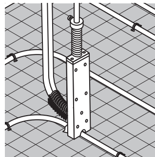
Zum Schluss die Systemrohre in dem berechneten Verlegeabstand auf die Tackerplatten auftackern.
