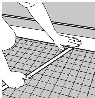
Die selbstklebende Folienschürze des Randdämmstreifens auf die Tackerplatte aufkleben
