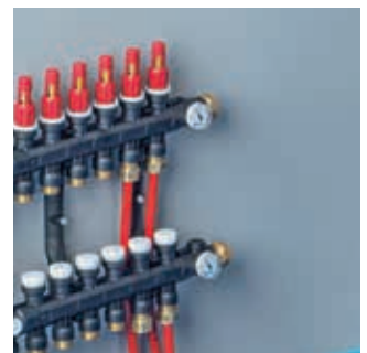
Die Uponor Nubos Systemrohre werden mittels Uponor Eurokonusverschraubungen 3/4" an den Heizkreisverteiler angeschlossen.
