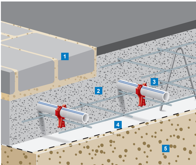
Beispielaufbau Uponor Meltaway Schnee- und Eisfreihaltung in Betonkonstruktion
