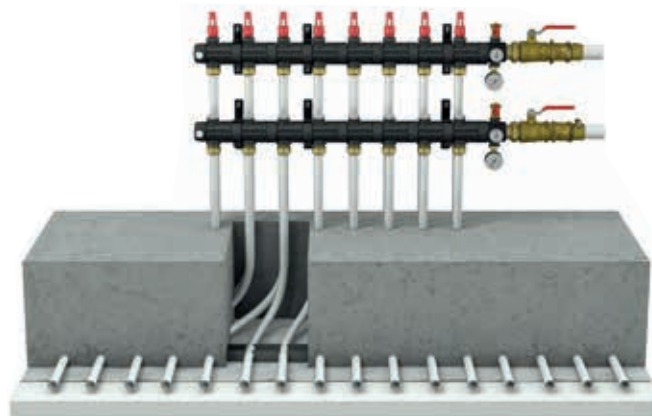
Heizkreisanschluss an den modularen Uponor Magna Industrierverteiler G 11/2"
